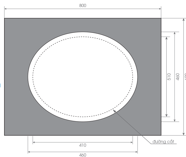
Bản vẽ cắt đá
